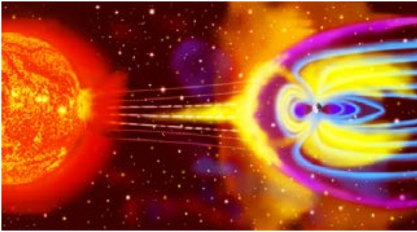
Обтекание магнитосферы Земли солнечным ветром
